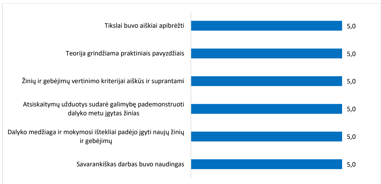
1 pav. Studijų programos Sistemų administravimas dalykų turinio kokybės vertinimas pagal šešis kriterijus (aritmetinis vidurkis)
